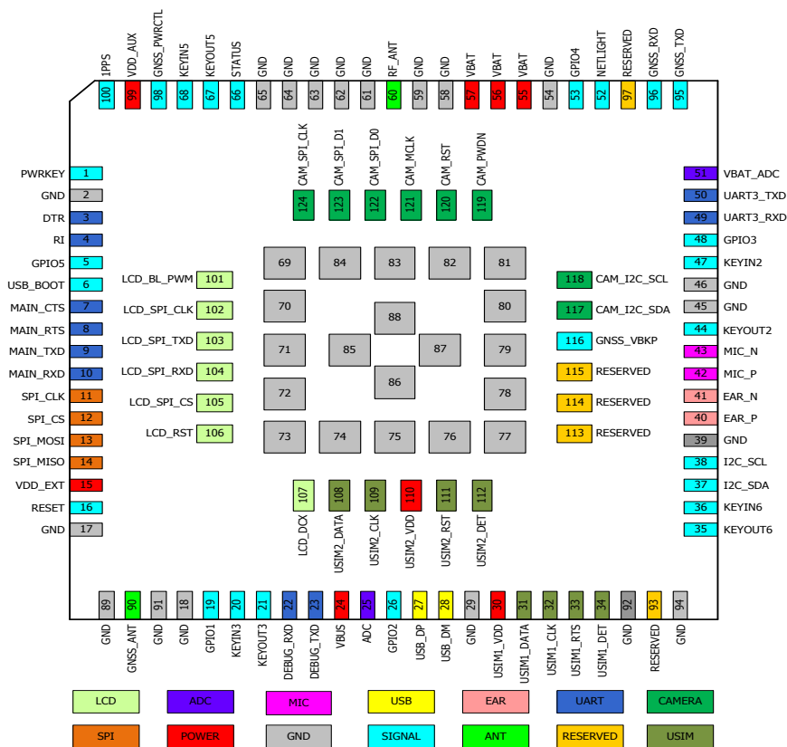
图 3-1 RHF4M603 模块管脚分布图（TOP 透视）
