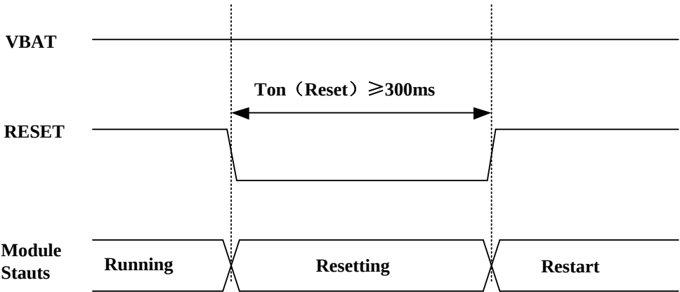
图 3-8 复位时序图
