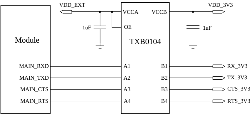
图 3-17 电平转换芯片电路
