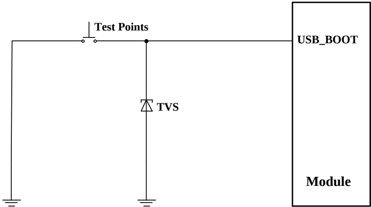
图 3-13 USB_BOOT 参考设计图
