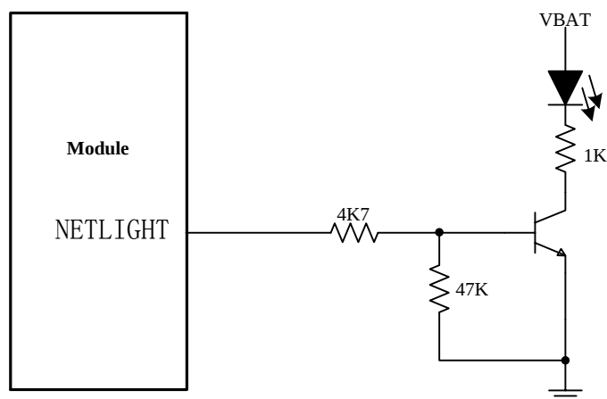
图 3-23 网络状态指示灯电路图
