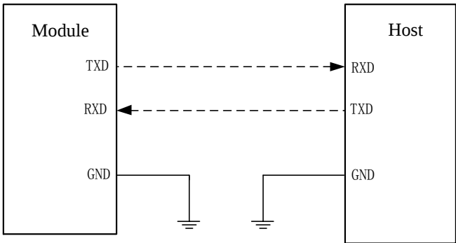
图 3-16 二线串口设计图
