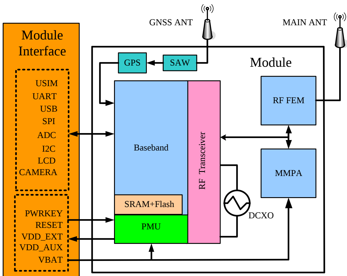
图 2-1 RHF4M603 模块功能框图
