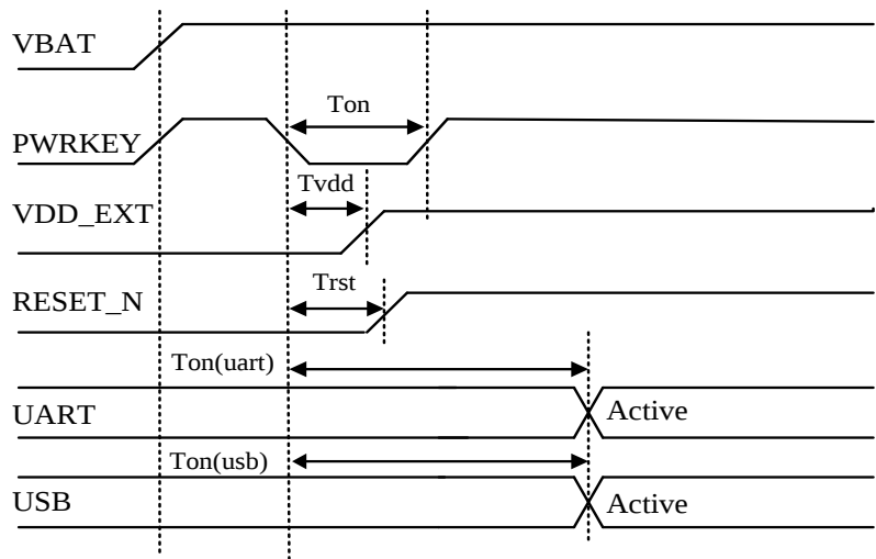
图 3-9 开机时序图
