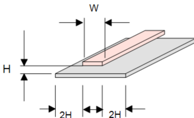
图 3-33 微带线的完整结构
