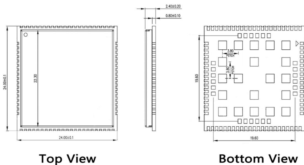
图 6-2 模块正视图与底视图(单位：毫米)
