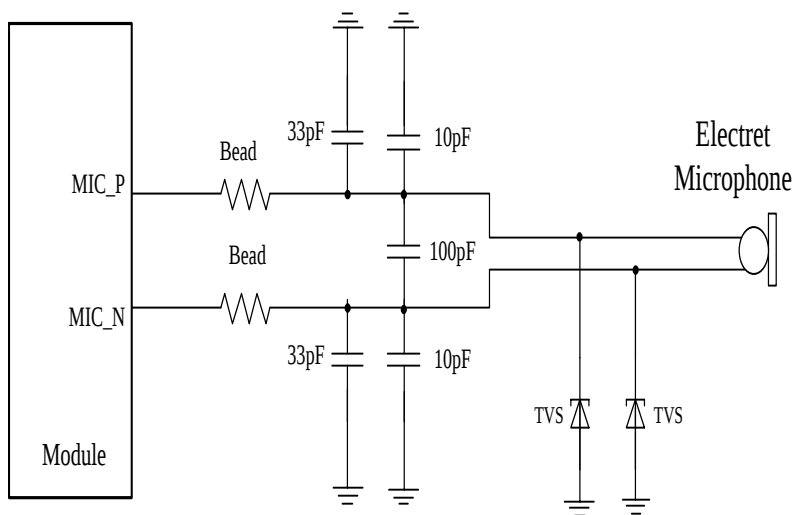
图 3-26 麦克风输入参考电路
