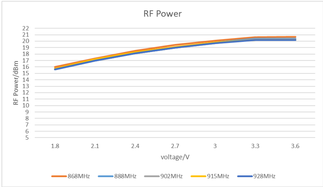
Figure 11 RF Power vs Voltage（868~928MHz）
